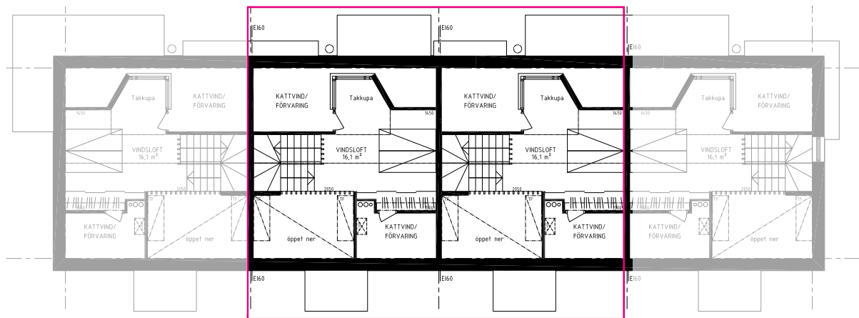
PLAN 3 (VINDSPLAN)
